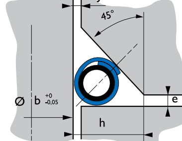
45° Type HN 140 - 240 (150 - 250)
