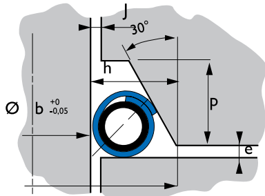
30° Type HN 140 - 240 (150 - 250)
