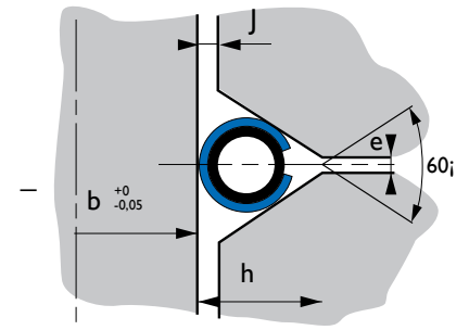
60° Type HN 100-200 (120-220)
